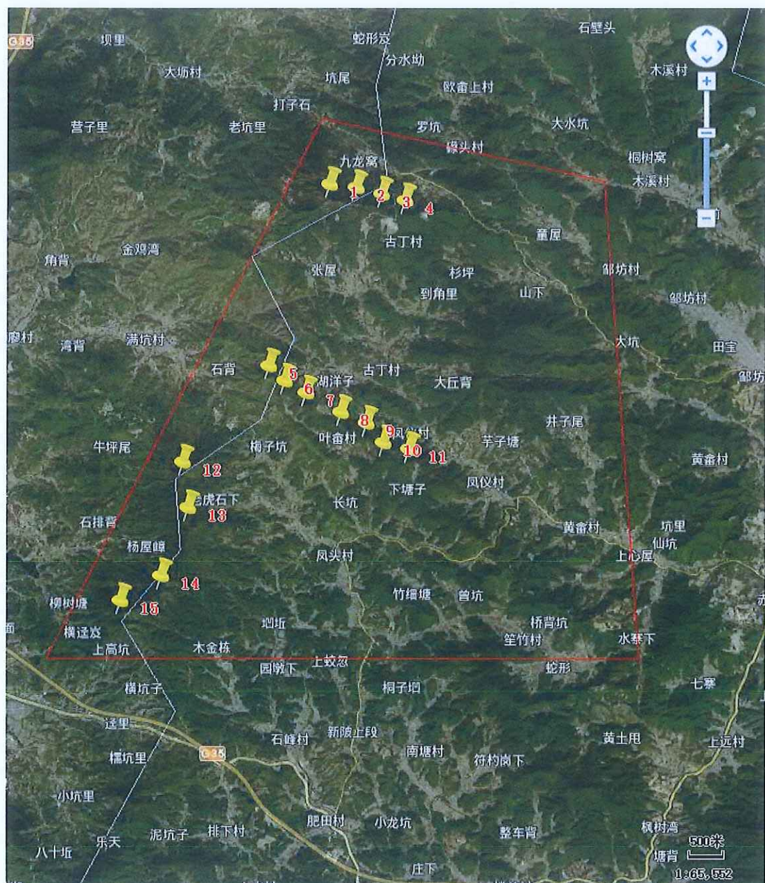
附图1 大华山风电场总平面布置图
